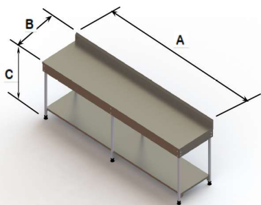
MESA DE ENCOSTO EM INÓX COM PRATELEIRA
