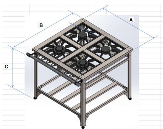
FOGÃO DE ENCOSTO
