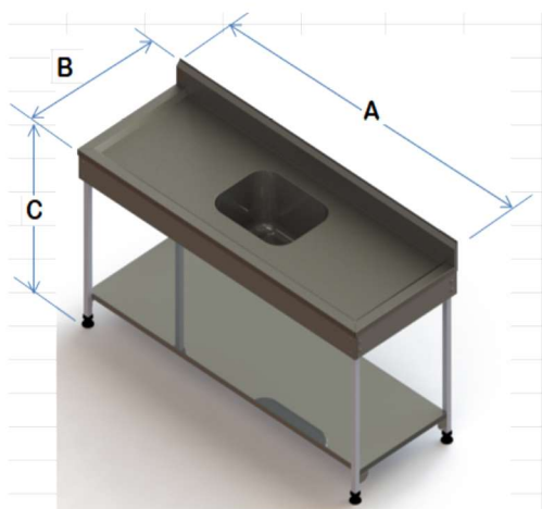
PIA DE ENCOSTO EM INÓX SEM PRATELEIRA
