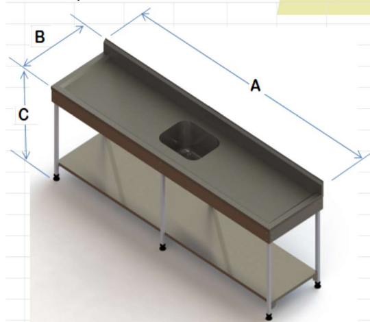
PIA DE ENCOSTO EM INÓX COM PRATELEIRA ( a partir de ( A ) 2000 mm, com 6 pés )
